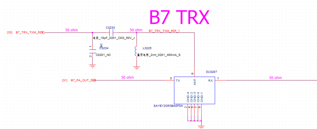
B7 Duplexer:
